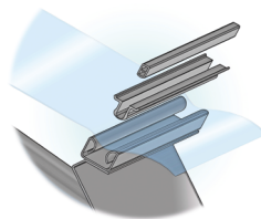
Richel-clips att fästa presenningen med och hålla den spänd och tät.
